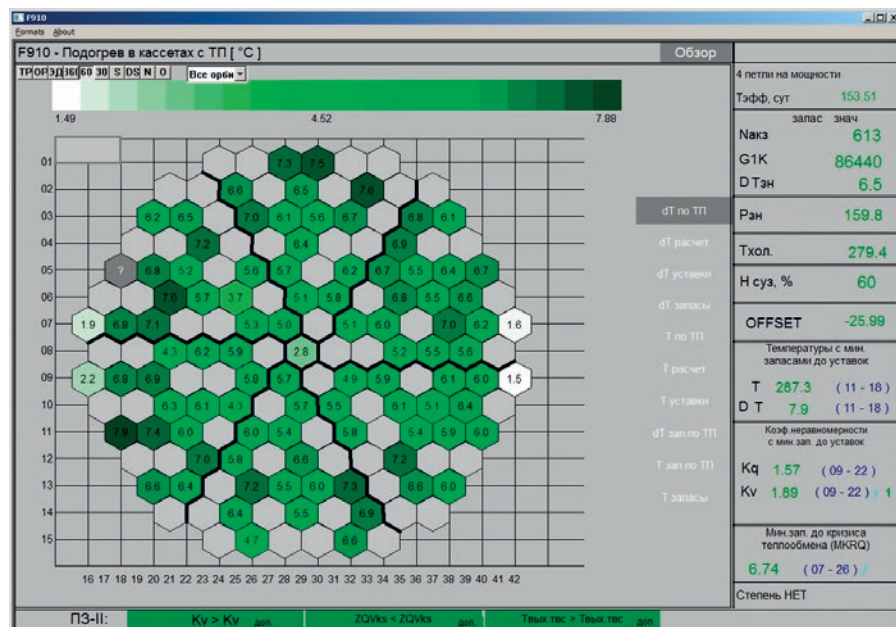
Фрагмент от видеокадър на активната зона на реактора
