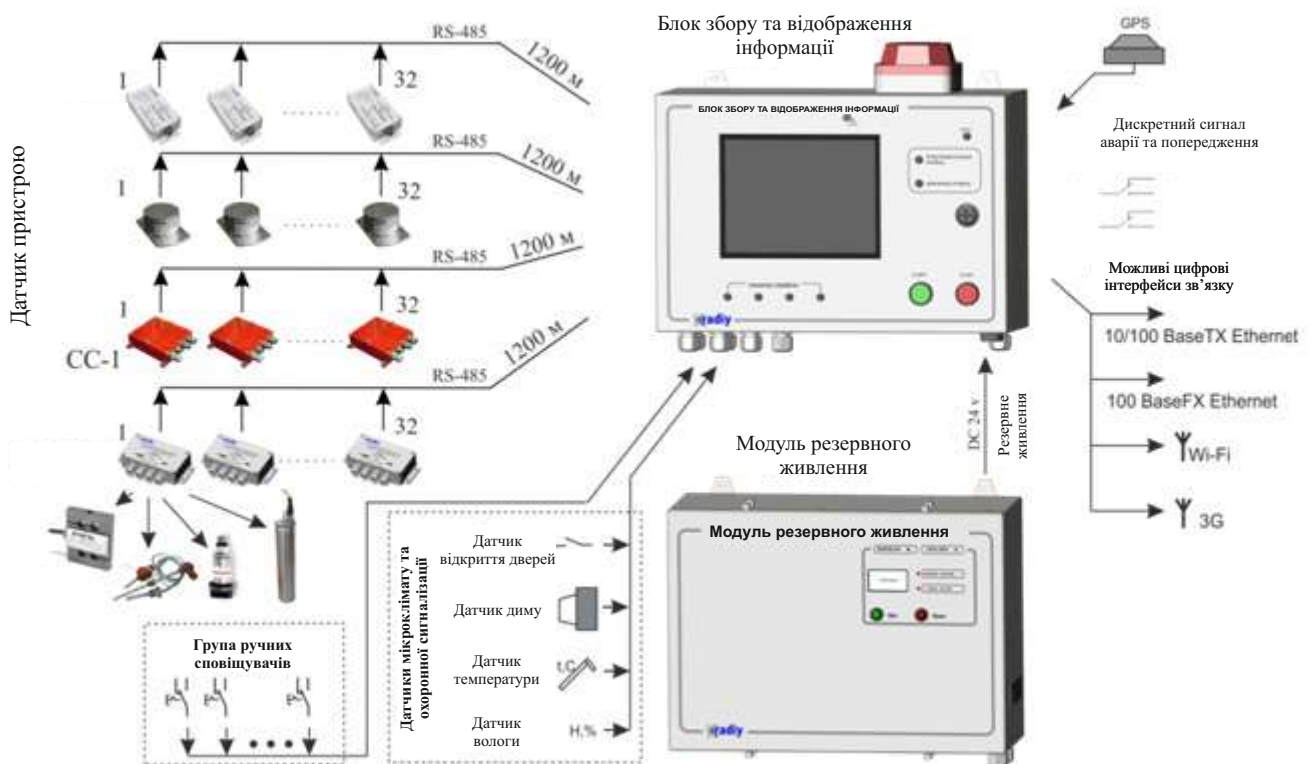
Мал. 1 Структурна схема сегмент АСРВ
