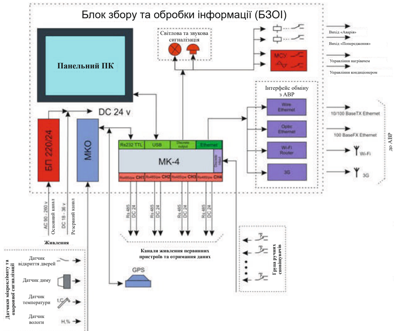
Мал. 3 Структурна схема взаємодії БЗОІ та периферії.
