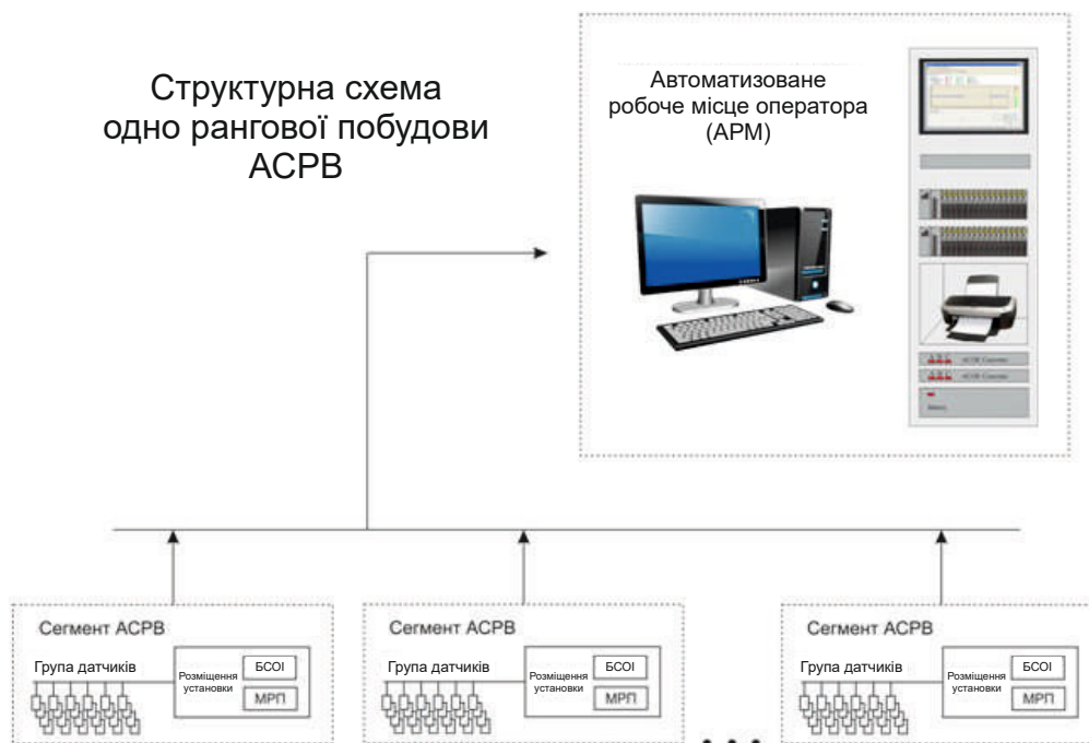
Мал. 2 Структурна схема побудови АСПВ як об'єднання однорангових сегментів.
