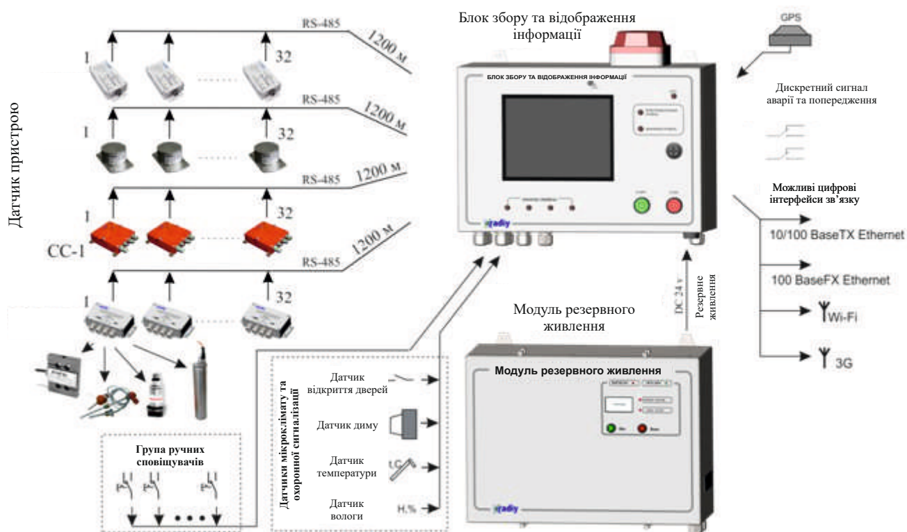
Мал. 1 Структурна схема сегменту АСРВ
